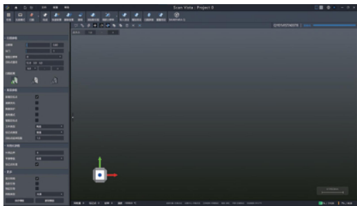
软件主界面
