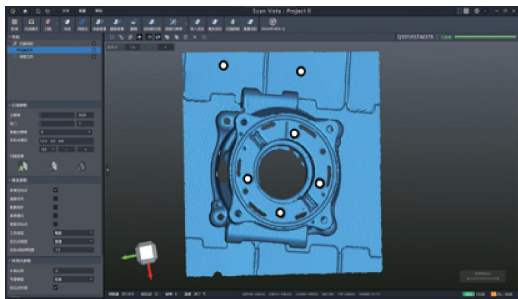
数据处理
